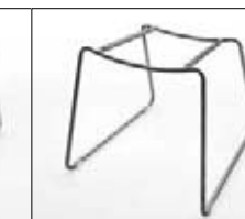
TEGE74AN Kufengestell Anthrazit lackiert B/H/T ca. 51 / 41 / 60 cm VPE: 2
